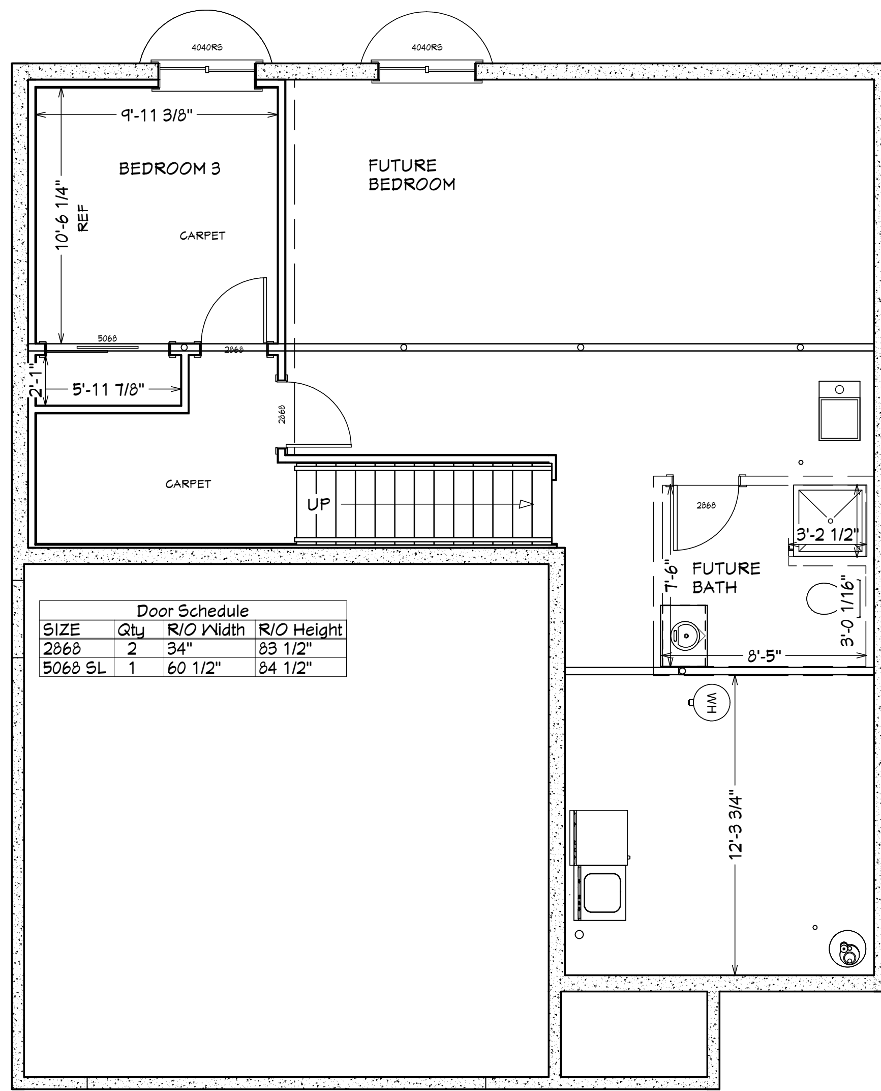
--BASEMENT PLAN--
