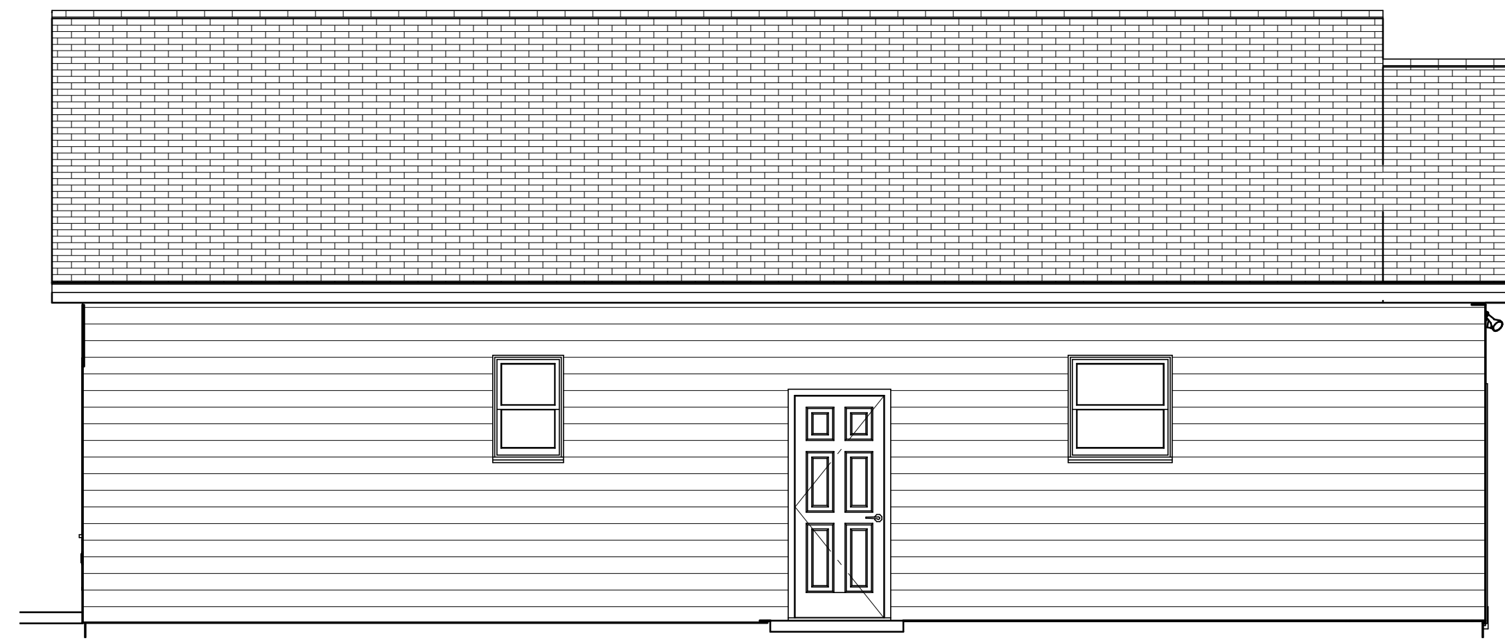
--LEFT ELEVATION--
